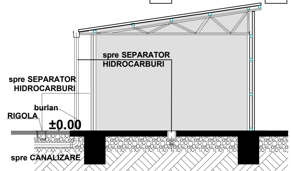
SECTIUNE TRANSVERSALA
