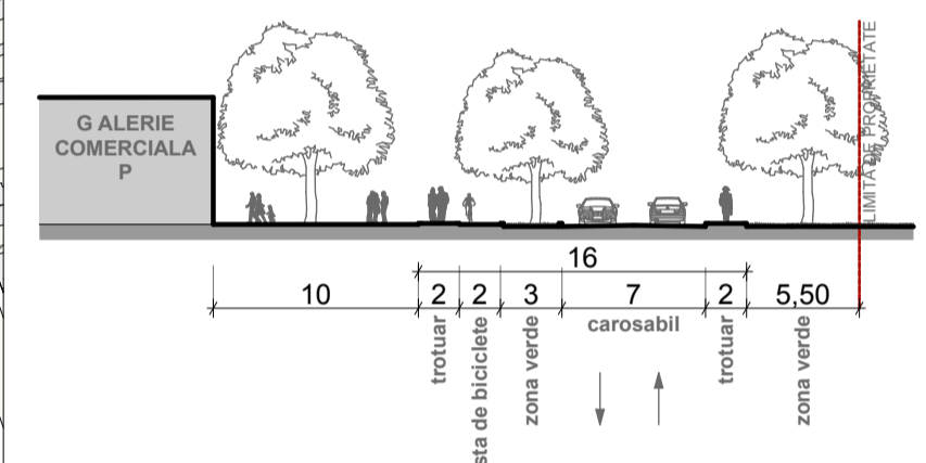
PROFIL TRANSVERSAL 2
