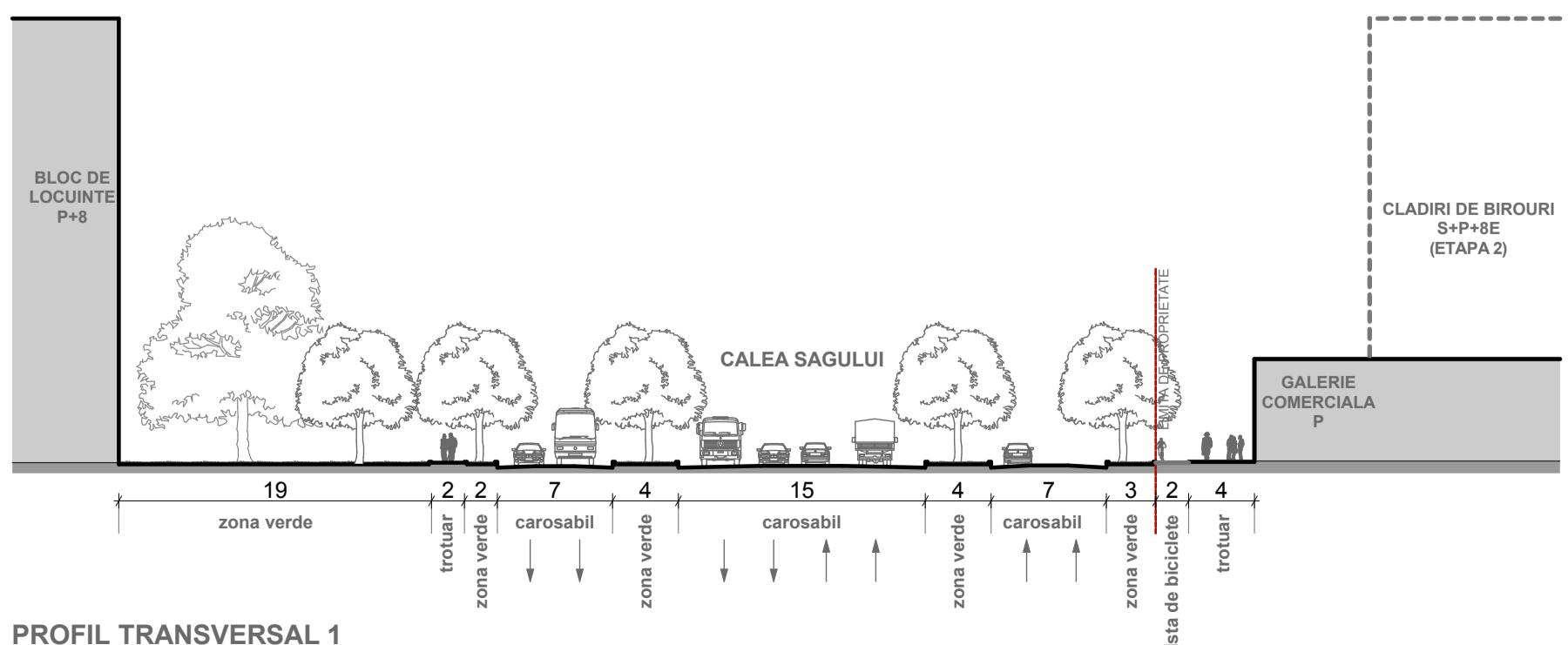
PROFIL TRANSVERSAL 1
