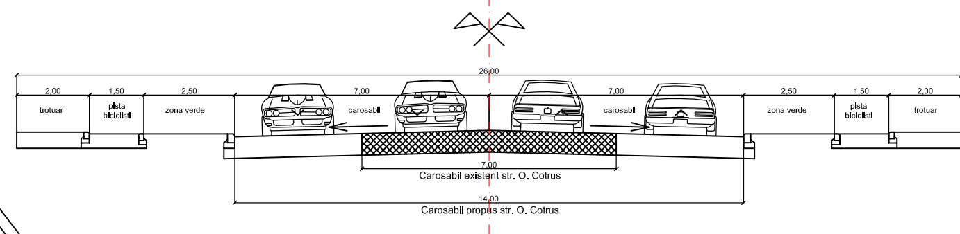
PROFIL TRANSVERSAL PROPUS STR. OVIDIU COTRUS Sc. 1:100
