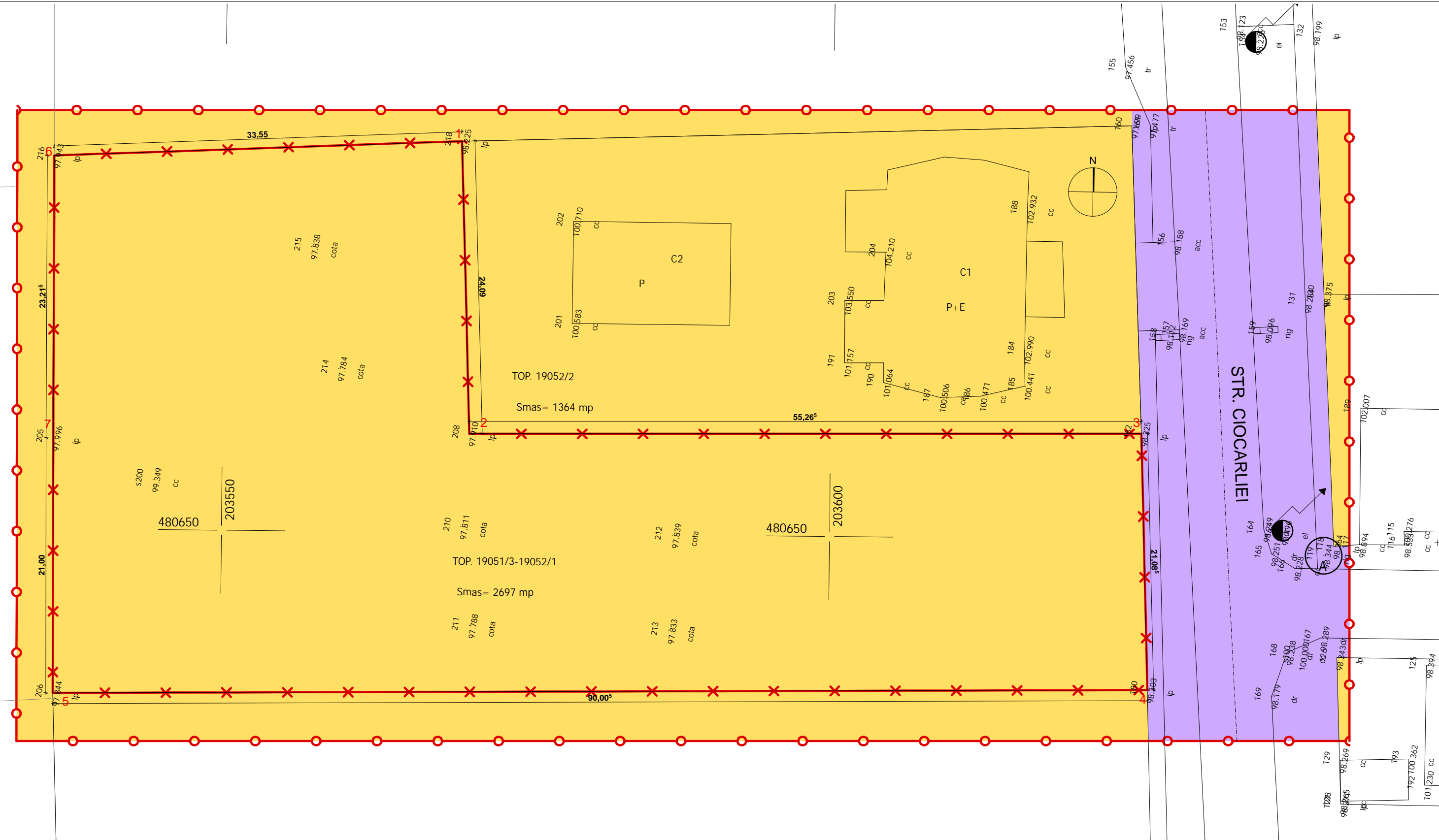
PUNCTE DE CONTUR ALE PARCELI 19051/3-19052/1 Sistemul de proiectie X, Y: STEREO '70
