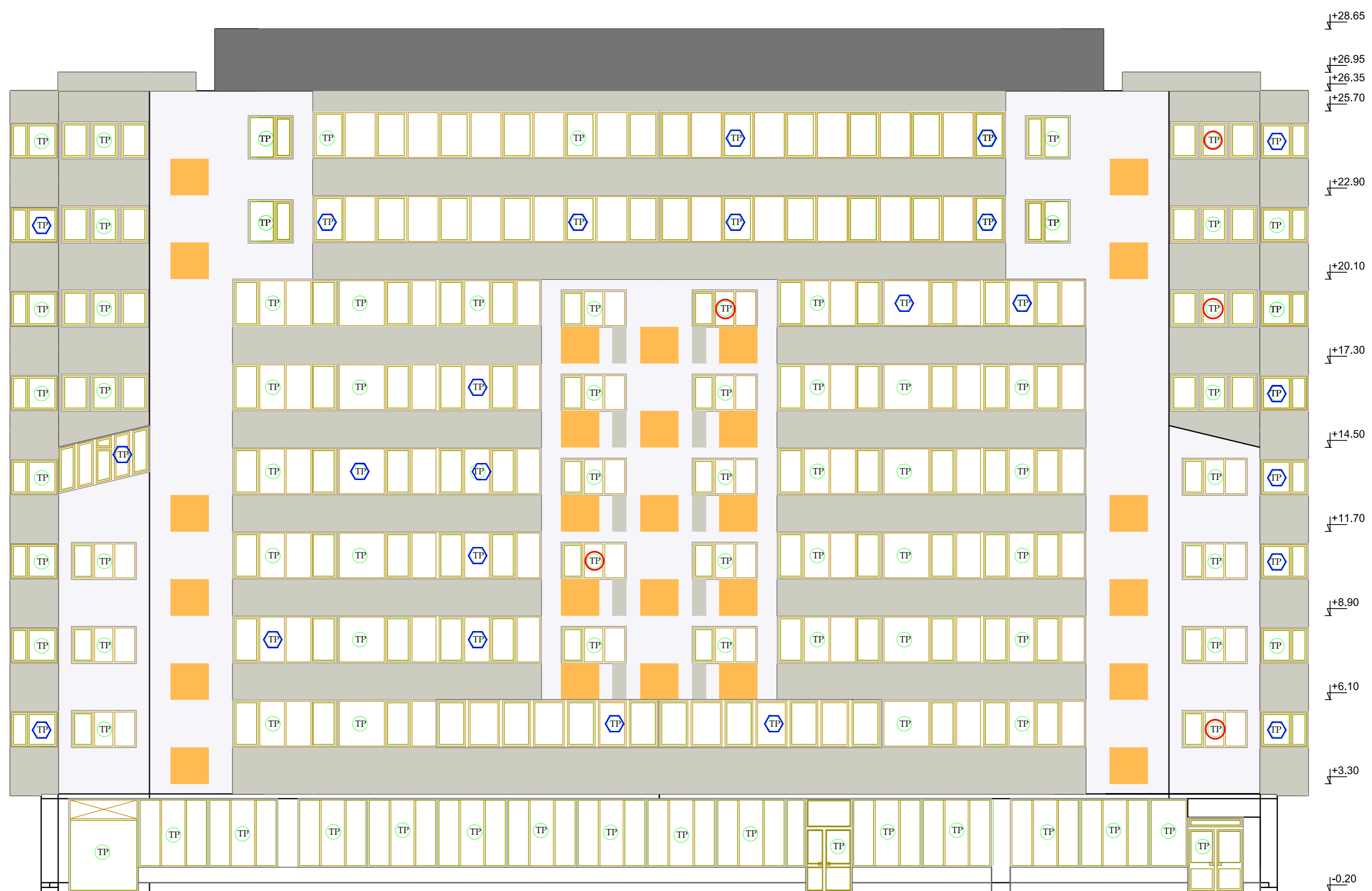
Fatada principala existenta Scara 1:100
