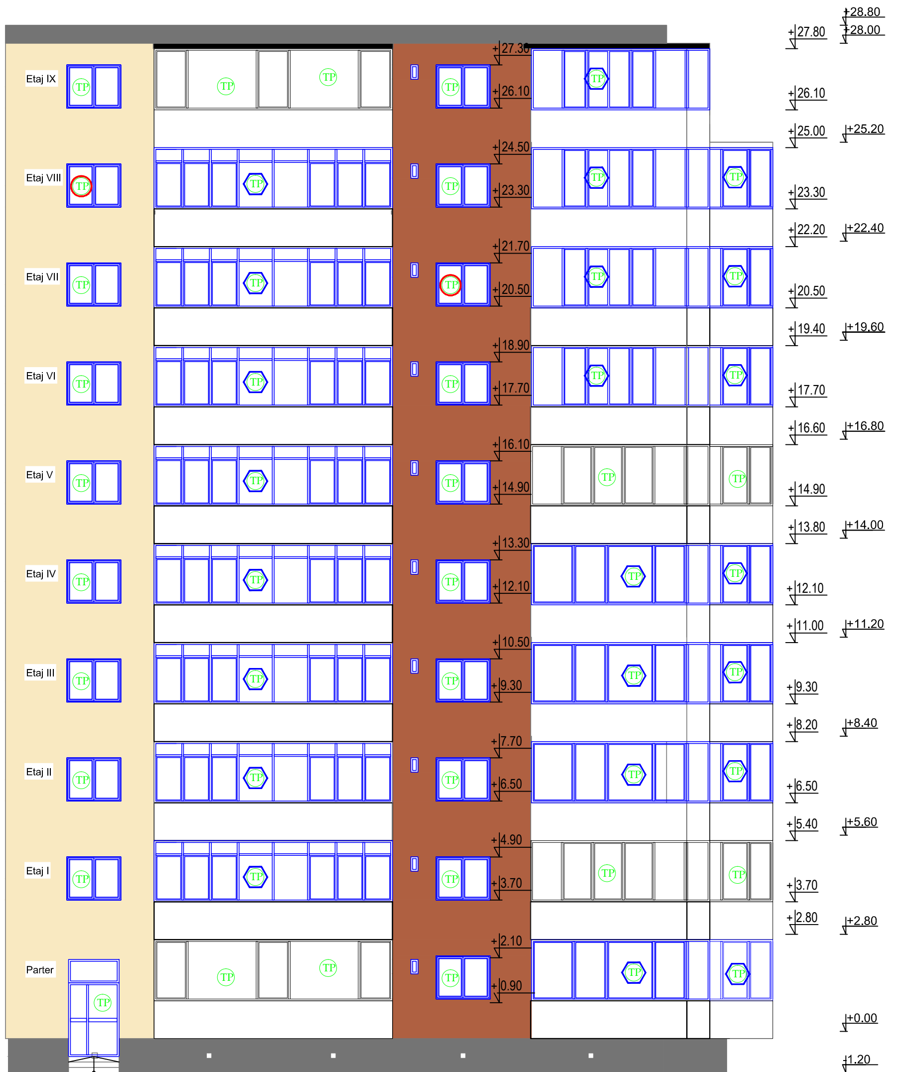
Fatada posteriora propusa Scara 1:100
