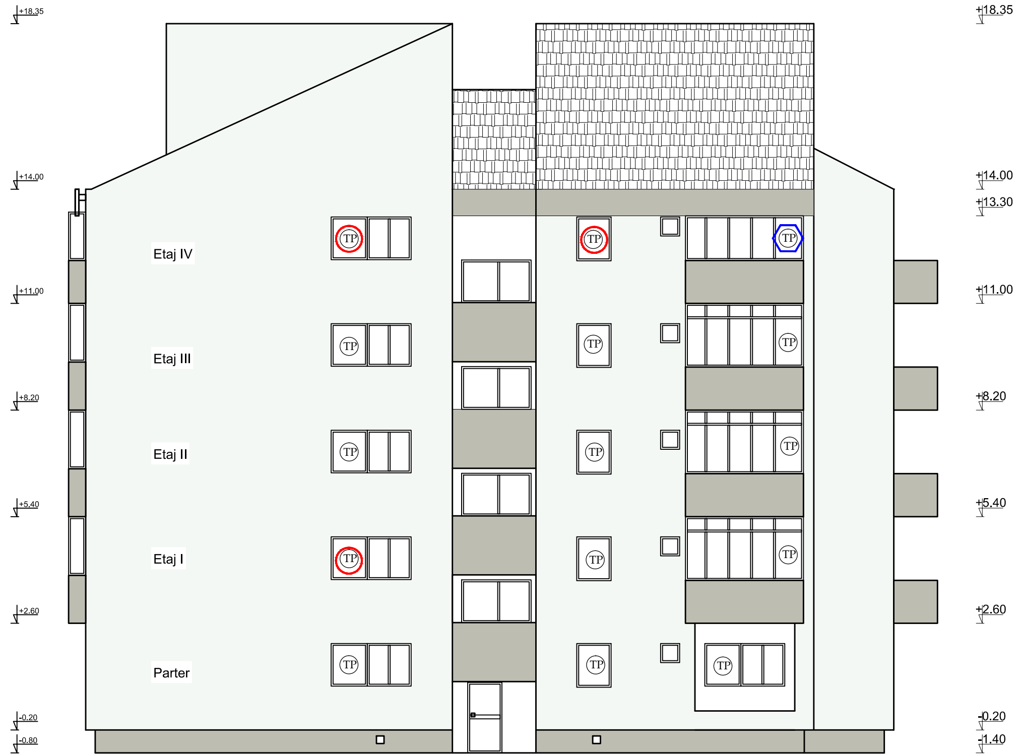
Fatada posterioara Scara 1:100
