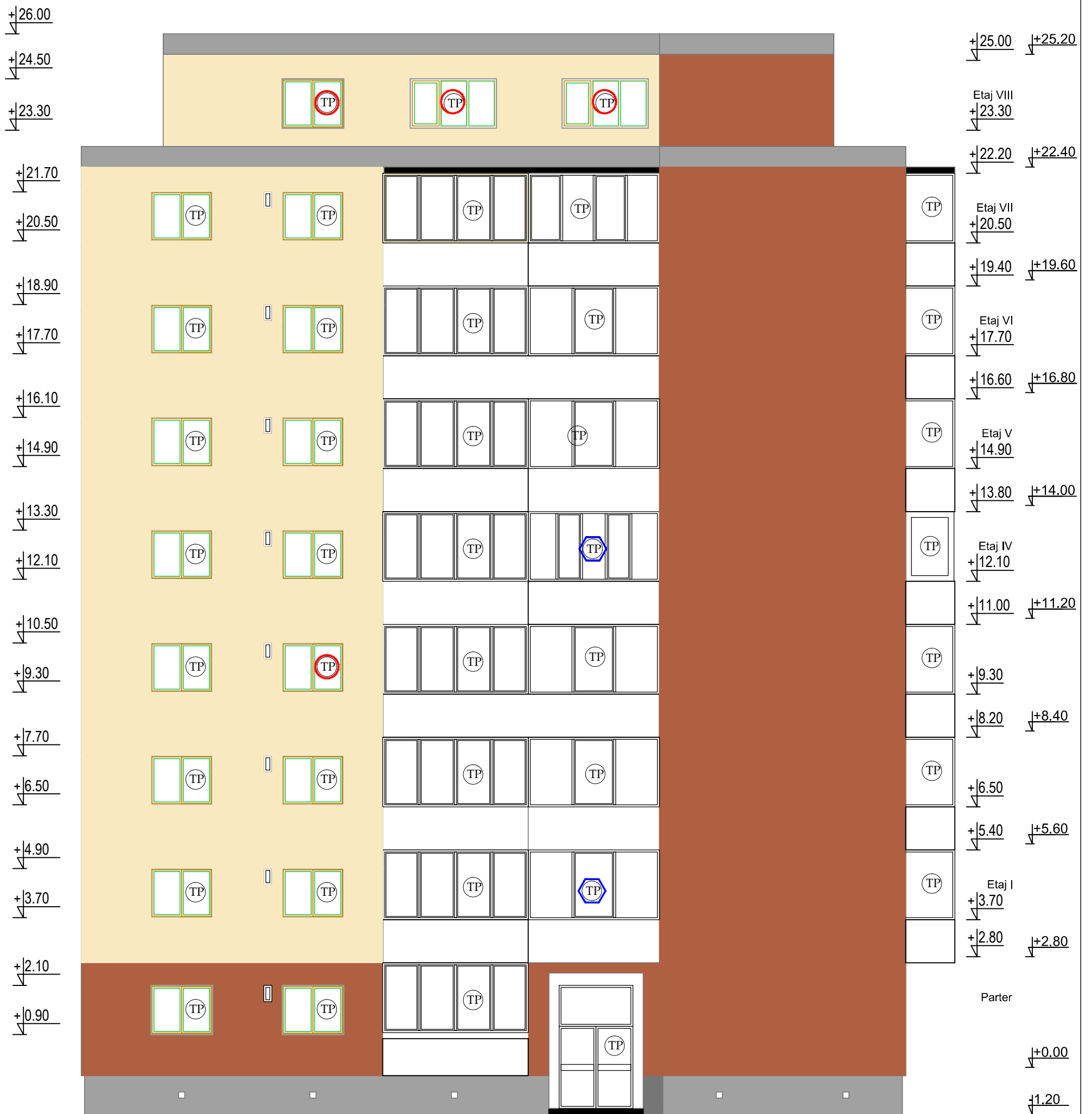
Fatada principala propusa Scara 1:100
