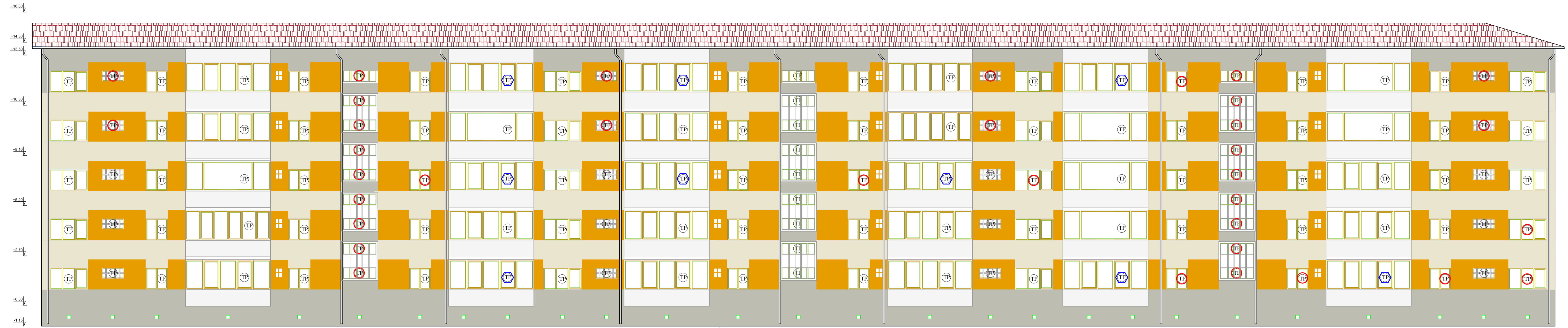
Fatada posterioara propusa
