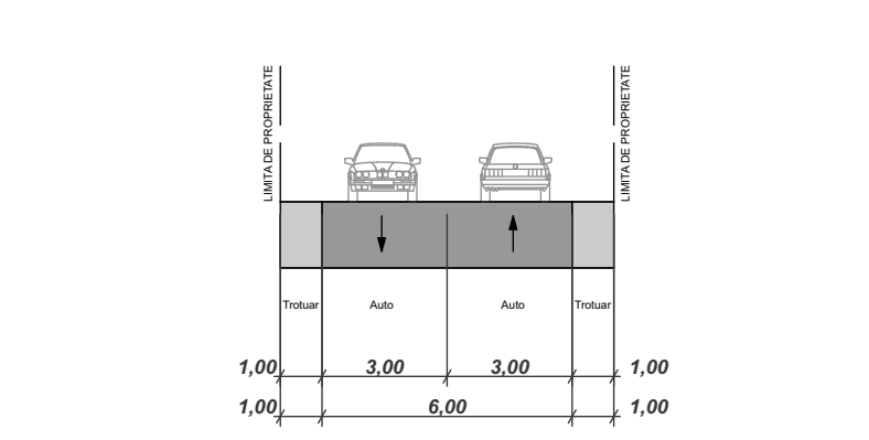
Profil Transversal PT2 - latime 8m
