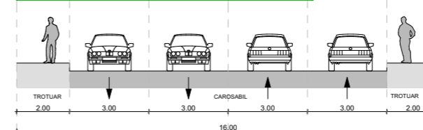
Profil Transversal A - lățime 16m
