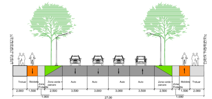
Profil Transversal 12 - lățime 27m
