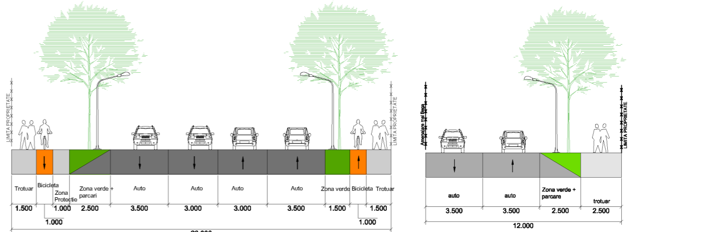
Profil Transversal 15 -lățime 23m
