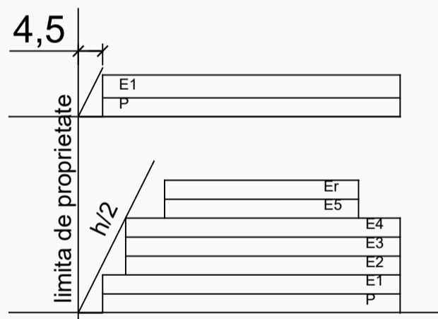
sectiuni caracteristice
