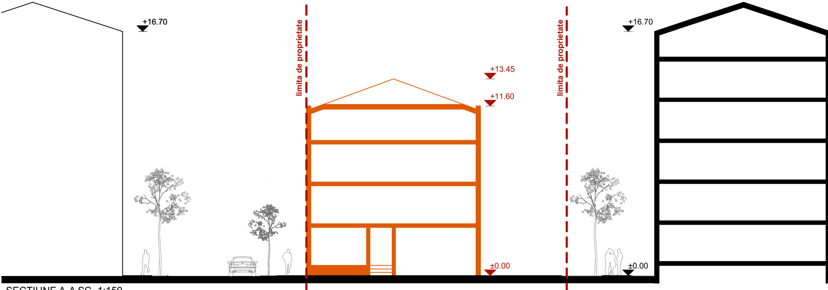
SECTIUNE A-A SC. 1:150
