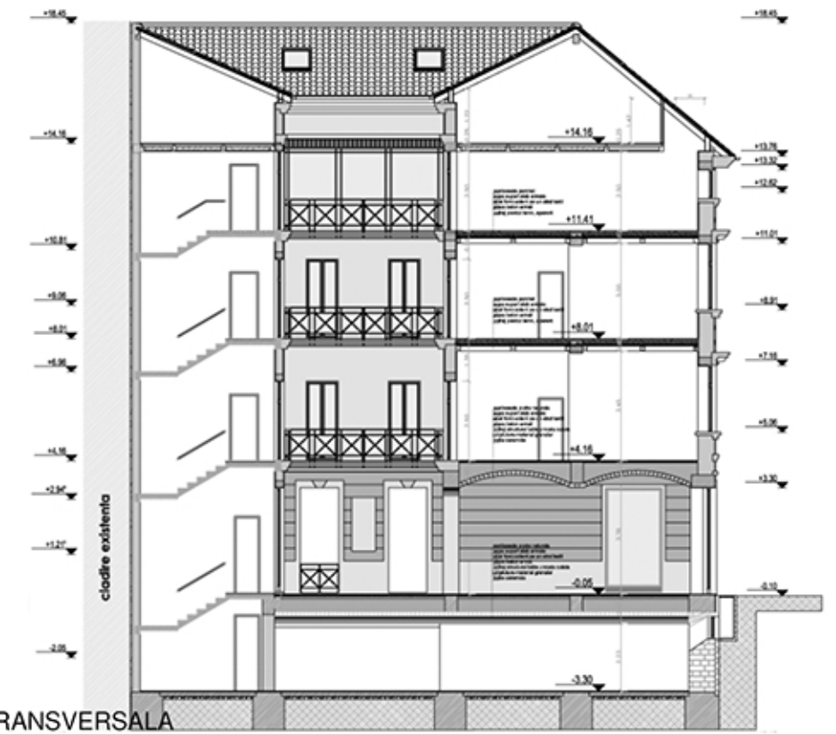
SECTIUNE LONGITUDINALA
