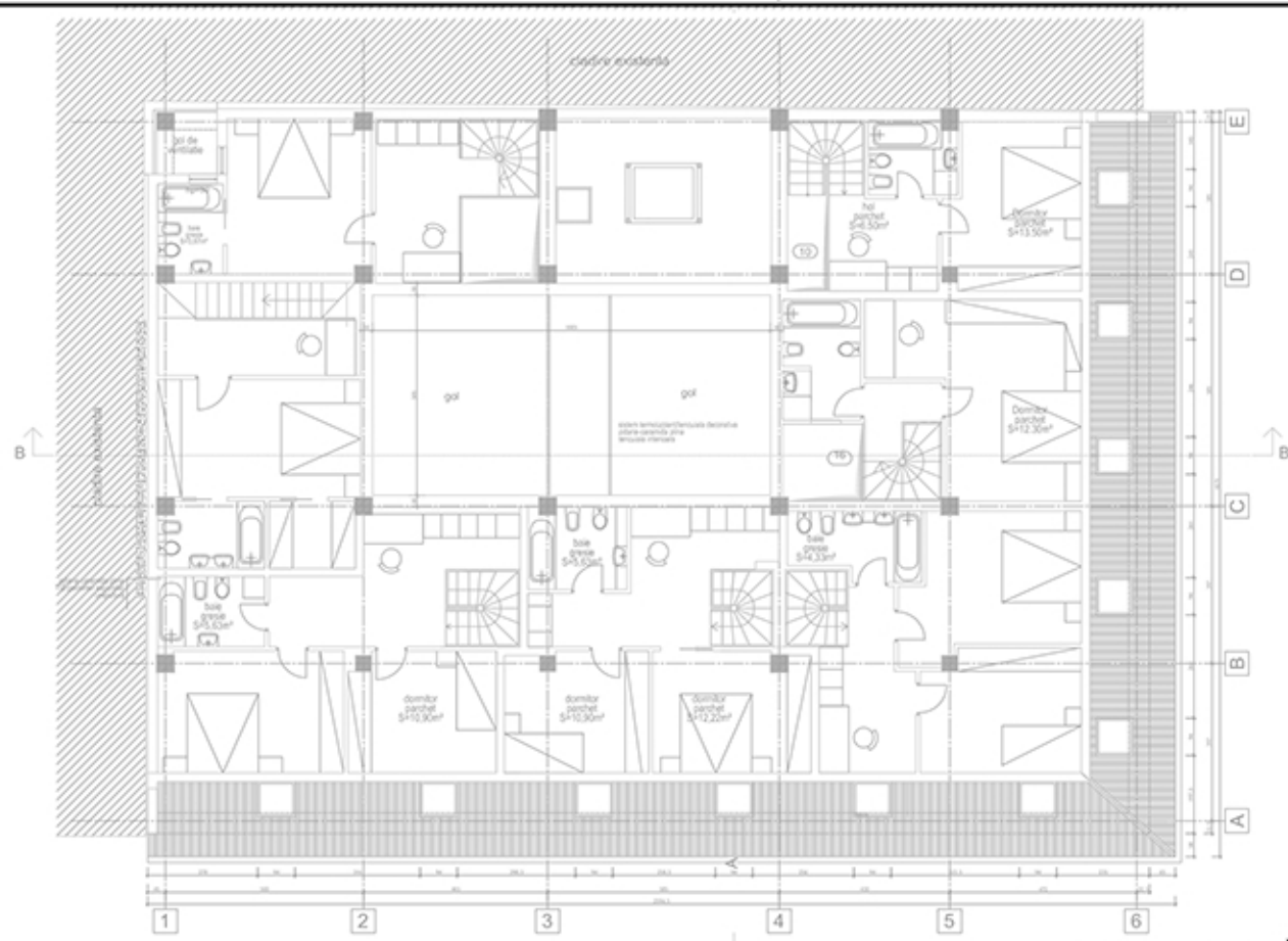
PLAN SUPANTĂ
