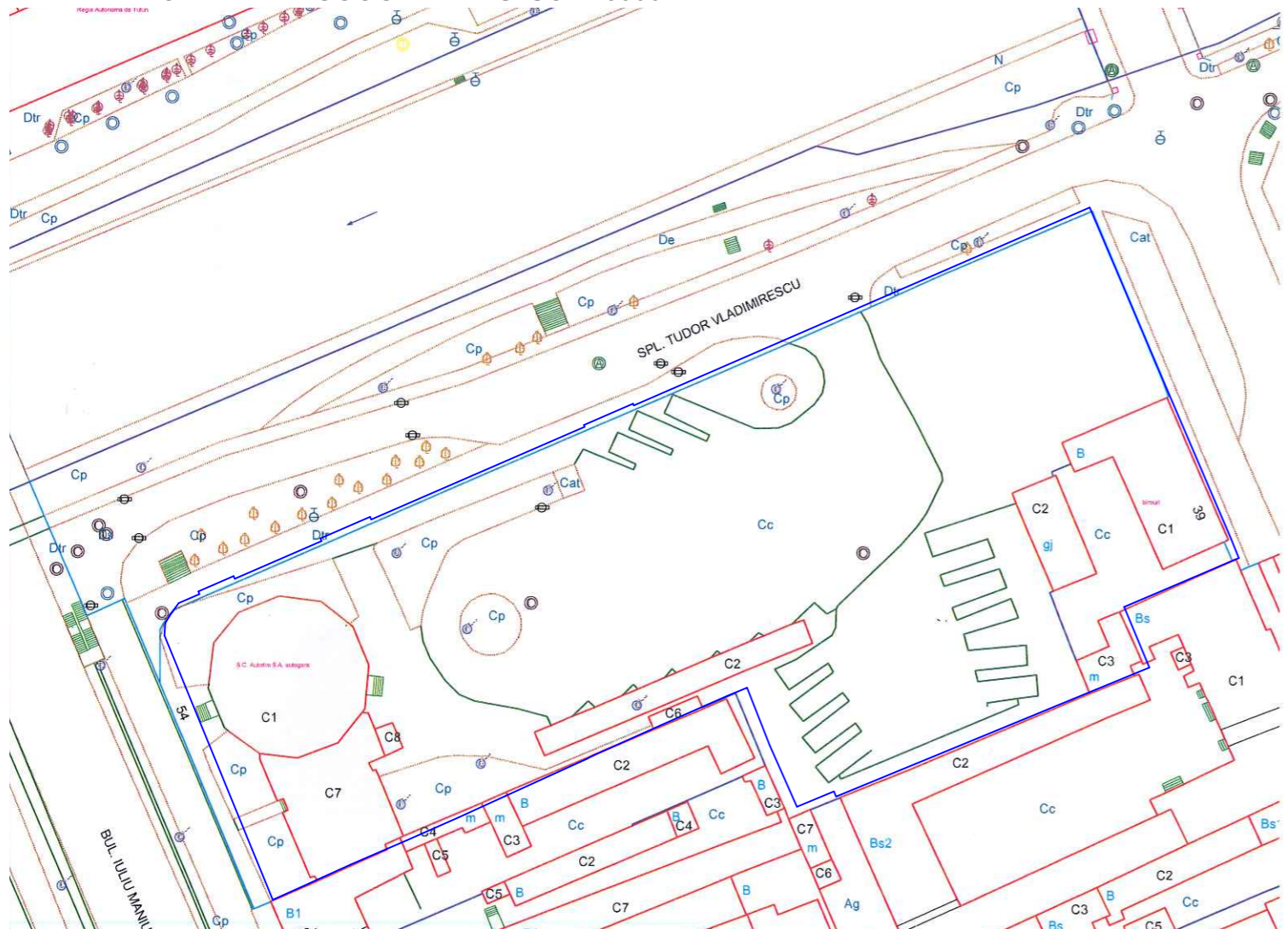
PLAN DE SITUATIE - PMT SC. 1 : 1000
