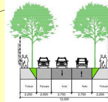
Profil Transversal 40 - lățime 12m Conform NOUL PUG - ETAPA 3, REVIZIA 3
