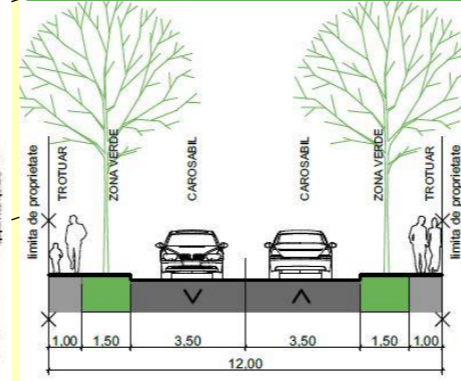
PTT 1 propus - latime 12m
