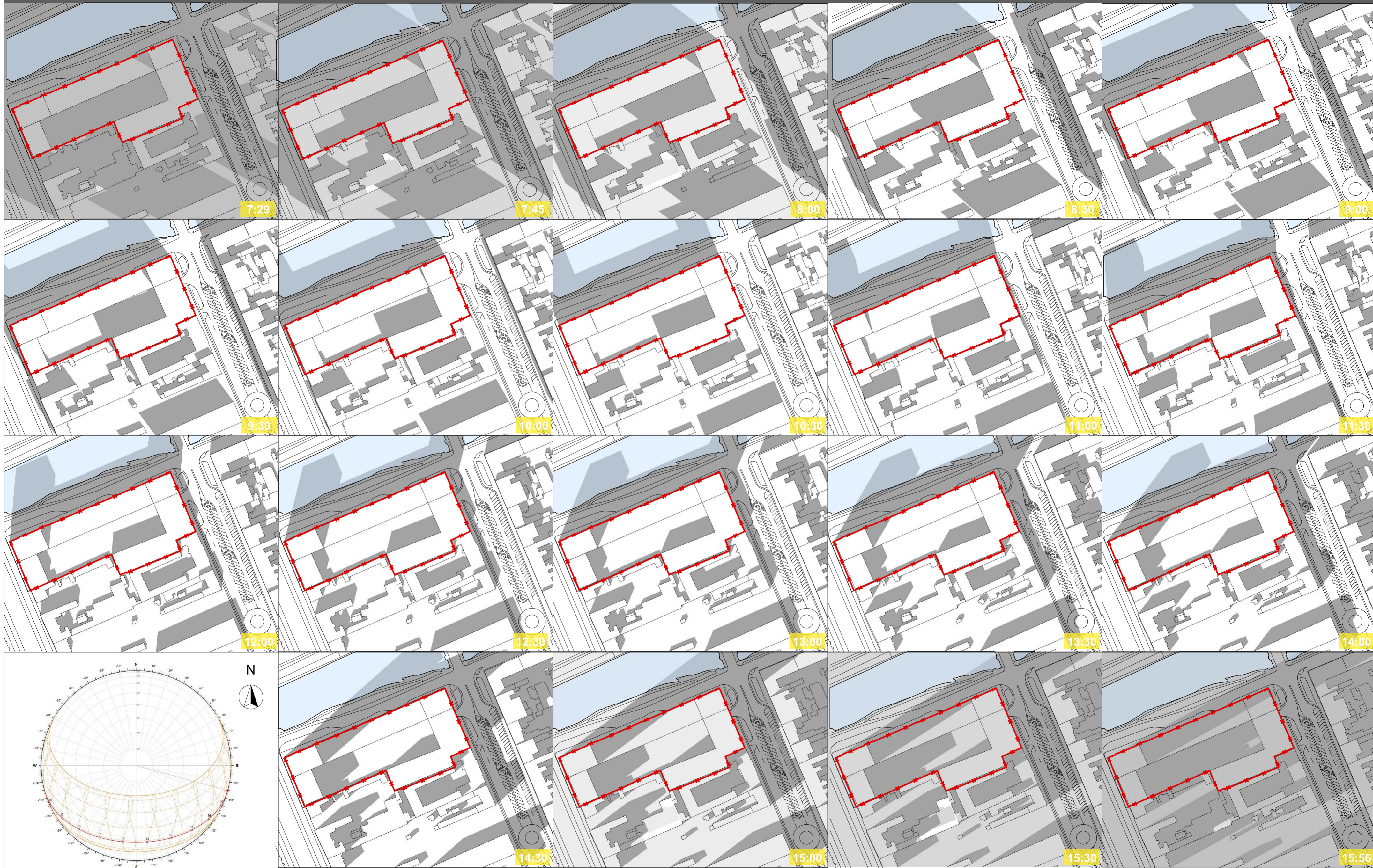
DIAGRAMA SOLARA TIMISOARA, SPLAIUL TUDOR VLADIMIRESCU 45°44'44.7" LATITUDINE NORDICA 21°12'24.5" LATITUDINE ESTICA RASARIT SOARE: 07:29 APUS SOARE: 15:56
