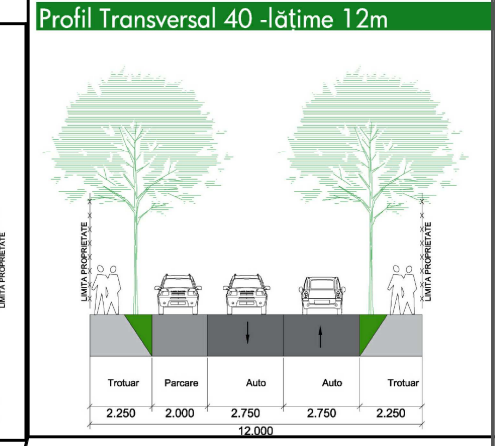
PROFILE TRANSVERSALE EXTRASE DIN PUG NOU IN LUCRU
