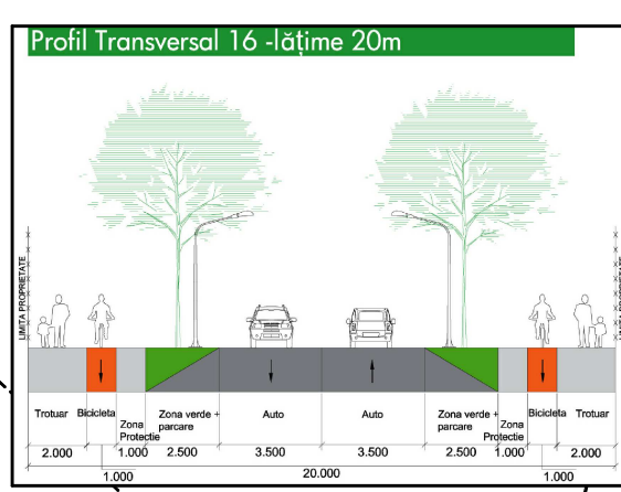
PROFILE TRANSVERSALE EXTRASE DIN PUG NOU IN LUCRU
