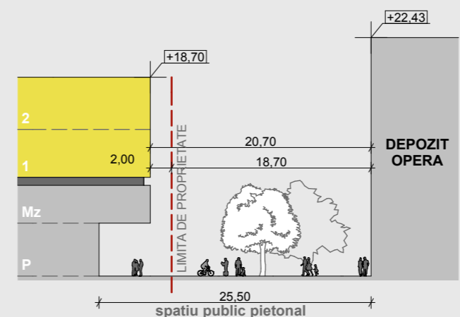
PROFIL STRADAL PP1 SC.1:500
