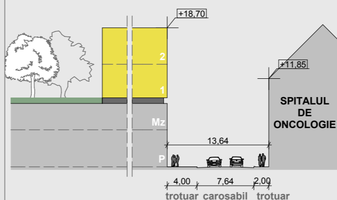
PROFIL STRADAL PP2 SC.1:500
