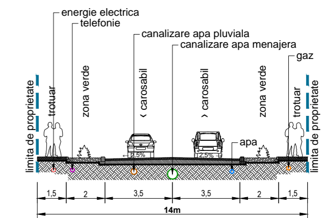
Profil transversal 2-2
