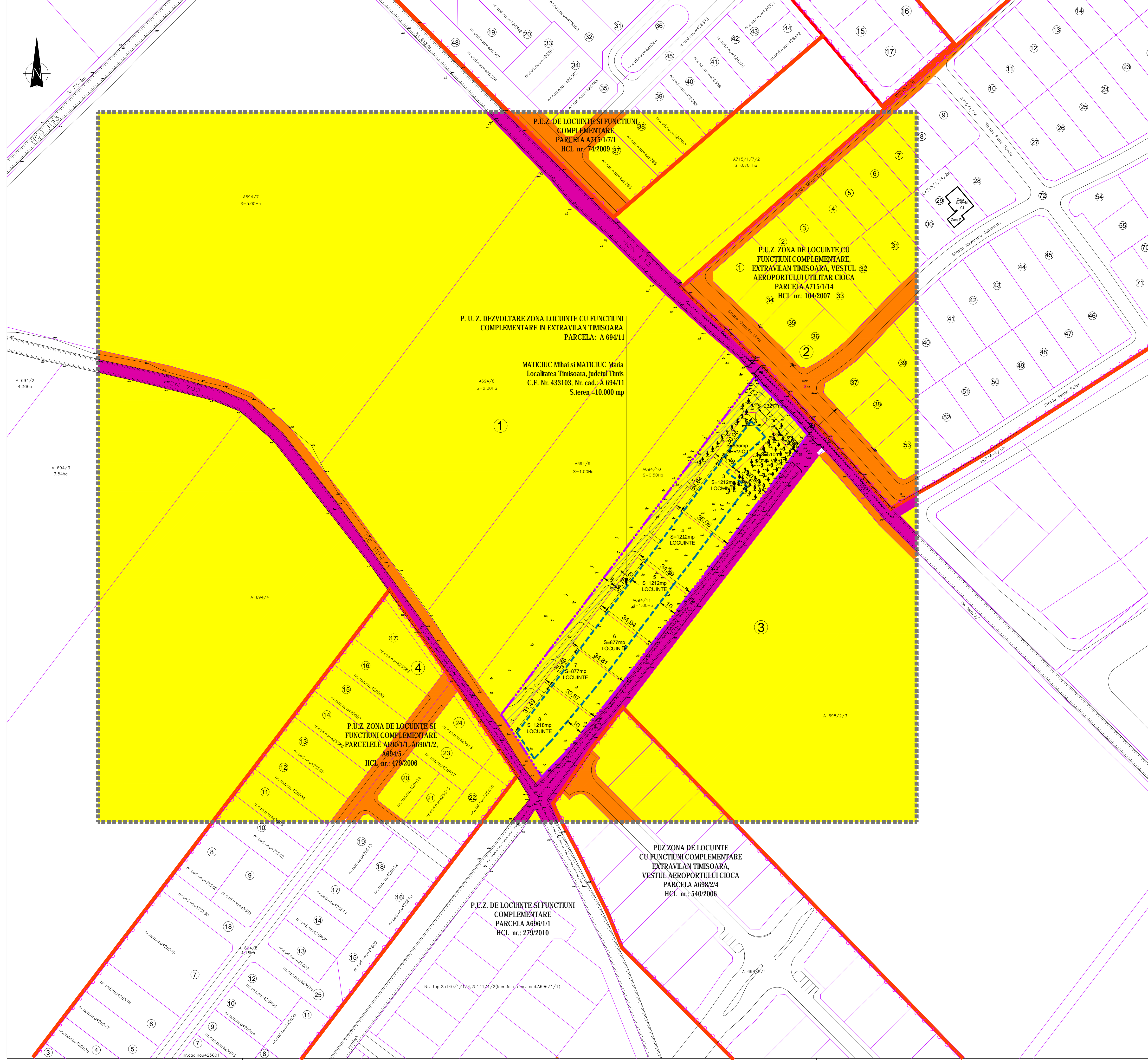
PLAN DE INCADRARE IN LOCALITATE sc. 1 : 5000
