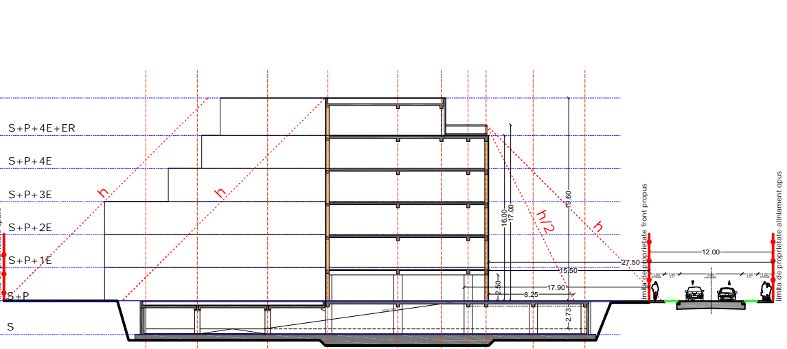
SECTIUNEA AA scara 1:500
