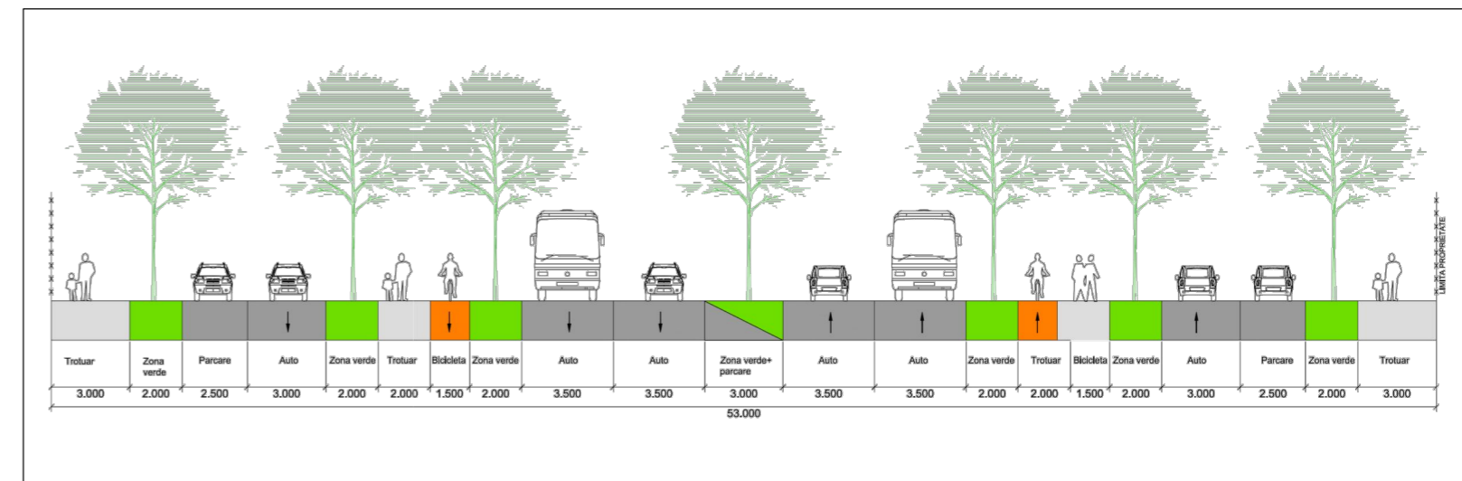
Profil transversal PT 23 (53m) - conform PUG Etapa 3
