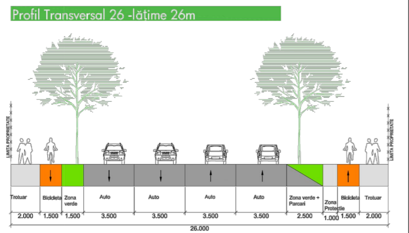
Profil transversal PT 26 - conform PUG Etapa 3
