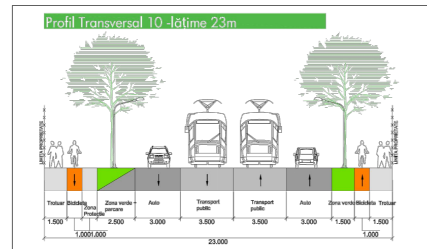
Profil transversal PT10 - conform PUG Etapa 3
