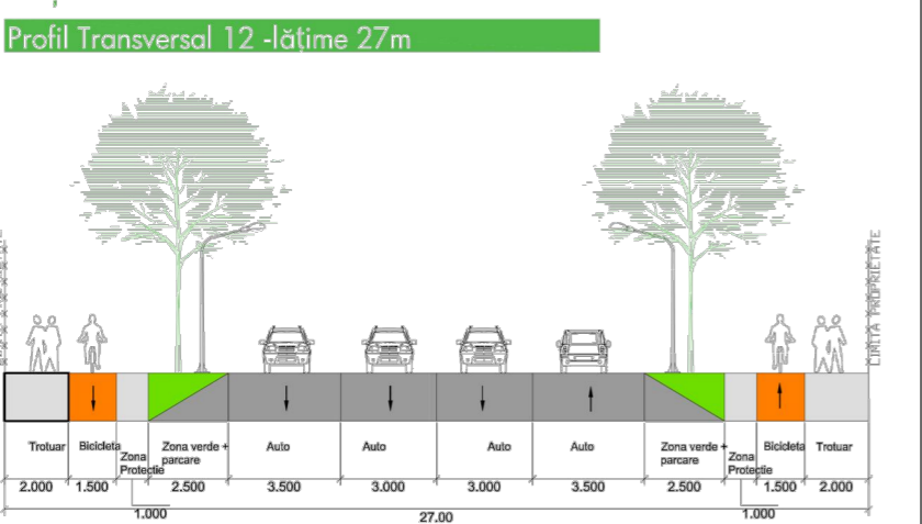
Profil transversal PT 12 - conform PUG Etapa 3
