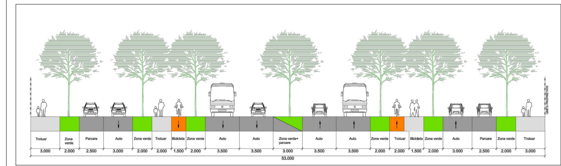
Profil transversal PT 23 (53m) - conform PUG Etapa 3
