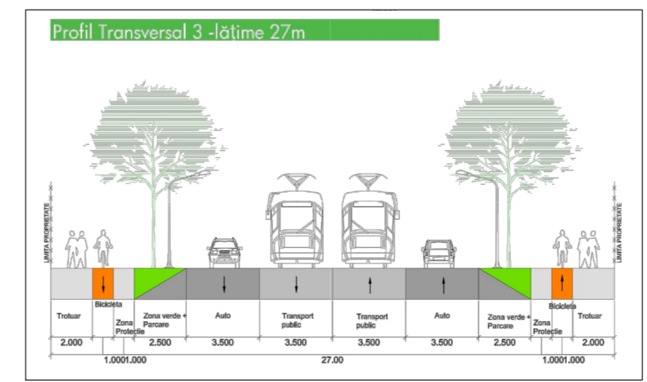
Profil transversal PT 3 - conform PUG Etapa 3
