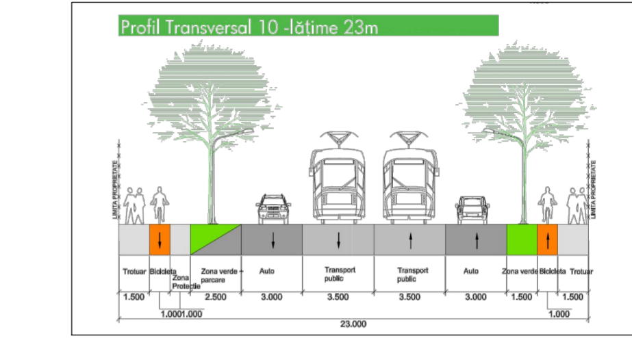
Profil transversal PT 10 - conform PUG Etapa 3
