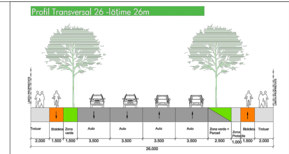
Profil transversal PT 26 - conform PUG Etapa 3
