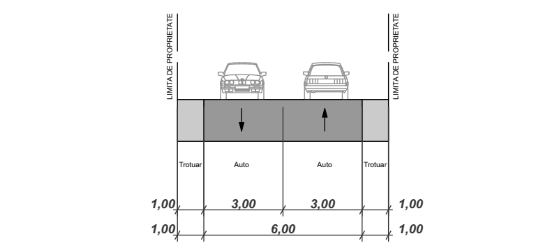
Profil Transversal PT2- latime 8m
