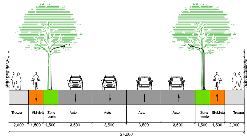
Profil Transversal 36 -lățime 24.5m
