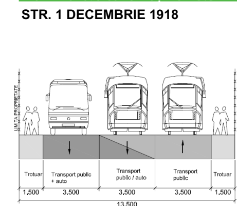
Profil Transversal 8 -lățime 13.5m
