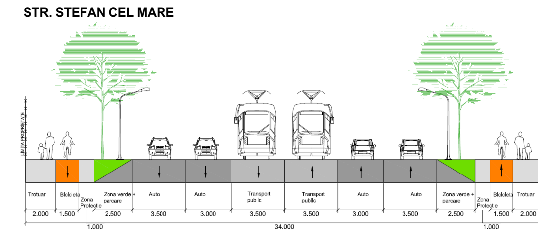
Profil Transversal 26 -lățime 26m
