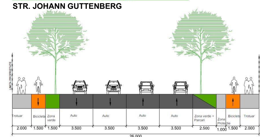
Profil Transversal 16 -lățime 20m
