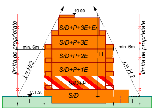
SECTIUNEA S1
