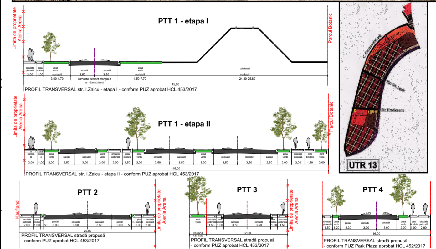
PROFILE TRANSVERSALE REGLEMENTATE SI MENȚINUTE PRIN DOCUMENTAȚII DE URBANISM APROBATE (tereunile afrente cailor de circulatiune nu reprezinta obiectul prezentei documentatii, vor fi menținute conform reglementarilor de urbanism aprobate)
