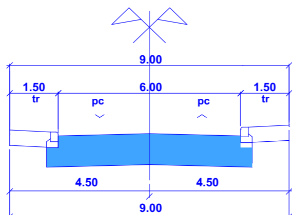
PROFIL TRANSVERSAL TIP PTT1
