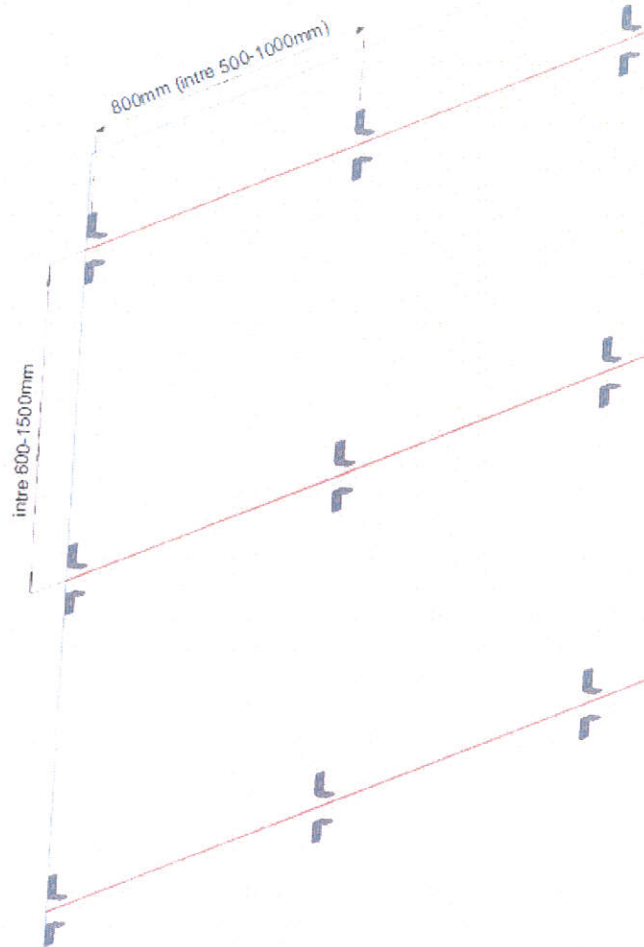
Detaliu vedere montare eclise pe perete Scara 1:10
