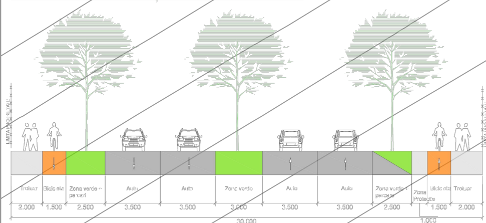
Profil Transversal 14 -lățime 30m
