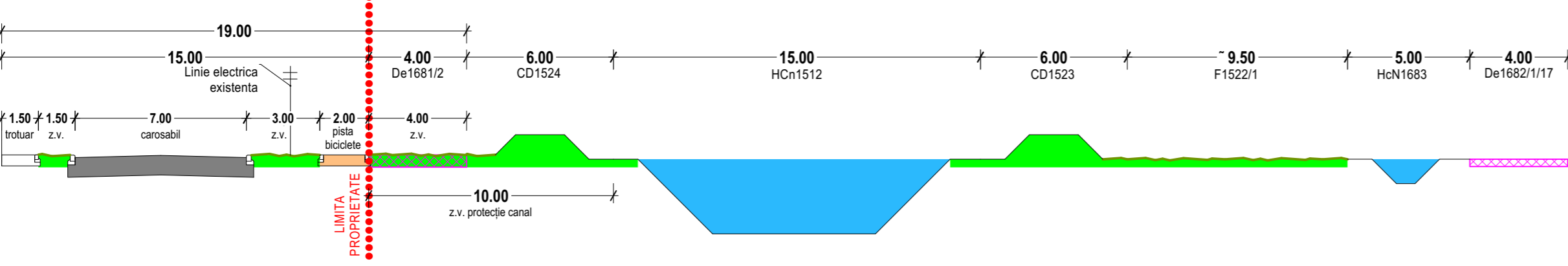
PROFIL TRANSVERSAL TIP PTT1 - DRUM COLECTOR PROPUS
