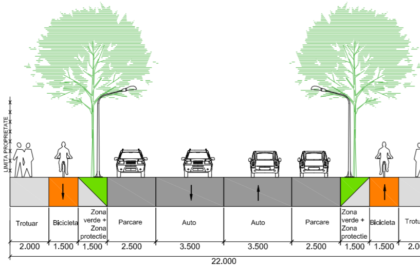
Profil transversal PTT 46 - 22 m lățime (Extras din PUG Timișoara propus în curs de avizare - Etapa 3 - prin H.C.L. 428/30.07.2013)
