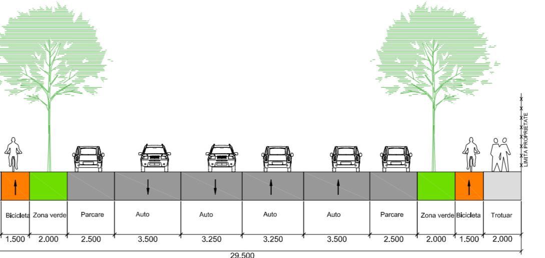
Profil transversal PTT 59 - 22,5 m lățime (Extras din PUG Timișoara propus în curs de avizare - Etapa 3 - prin H.C.L. 428/30.07.2013)
