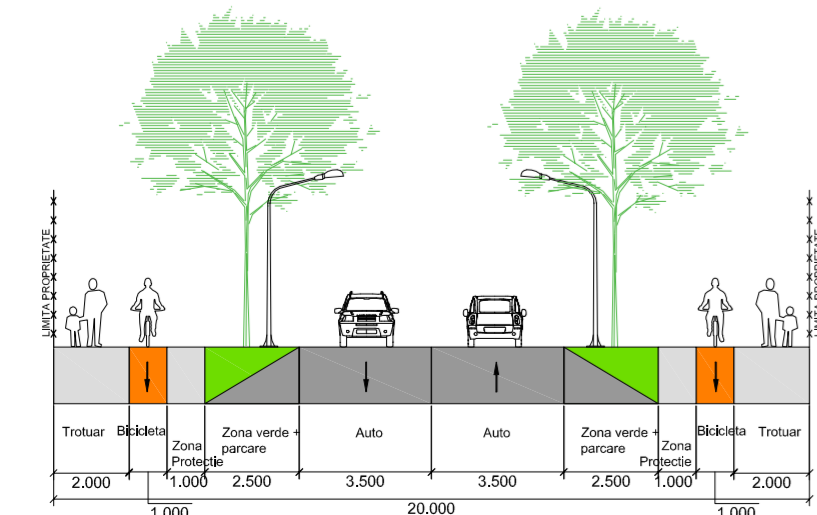
Profil transversal PTT 16 - 20 m lățime (Extras din PUG Timișoara propus în curs de avizare - Etapa 3 - prin H.C.L. 428/30.07.2013)
