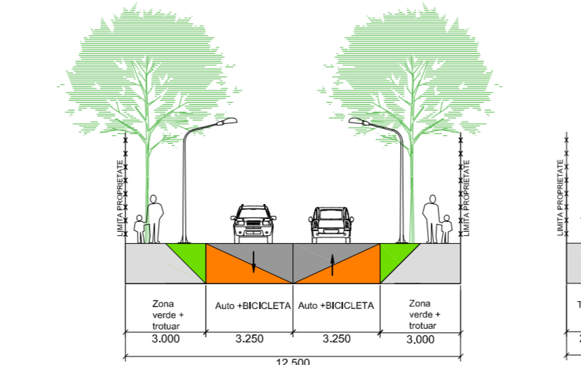
Profil transversal PTT 47 - 12,5 m lățime (Extras din PUG Timișoara propus în curs de avizare - Etapa 3 - prin H.C.L. 428/30.07.2013)
