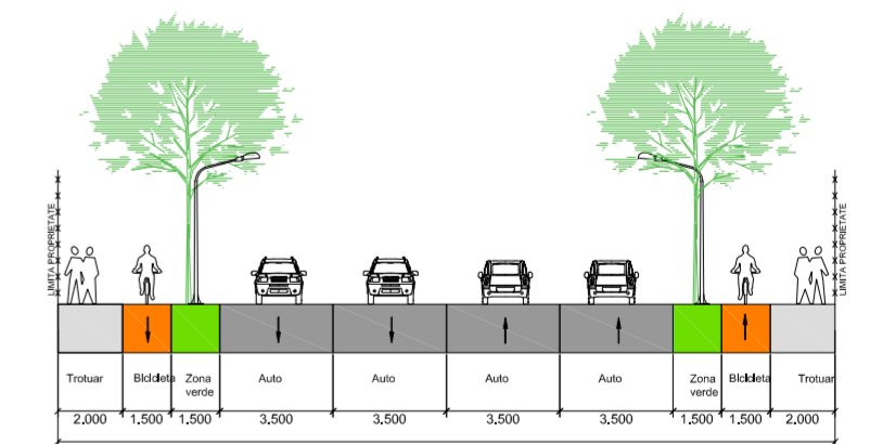
PTT70 : Profil stradal propus prin PUG (ETAPA 3, REVIZUA 3, ANEXA 6 PTT 70)
