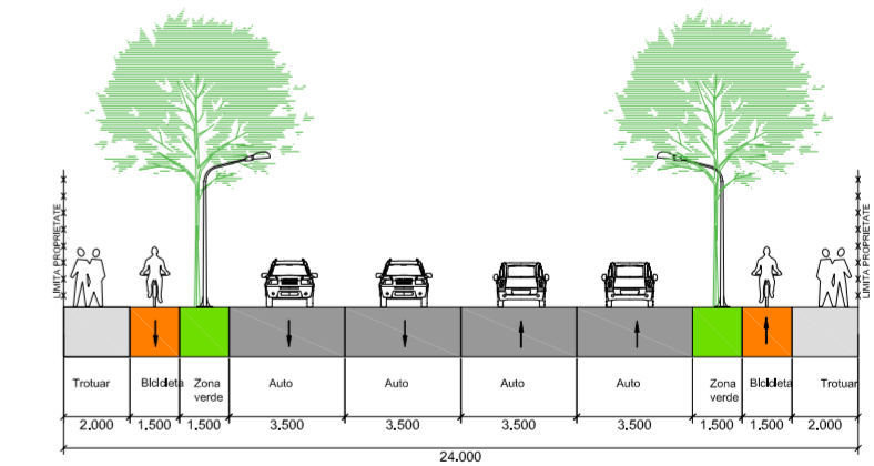
PTT70 : Profil stradal propus prin PUG (ETAPA 3, REVIZIA 3, ANEXA 6 PTT 70)
