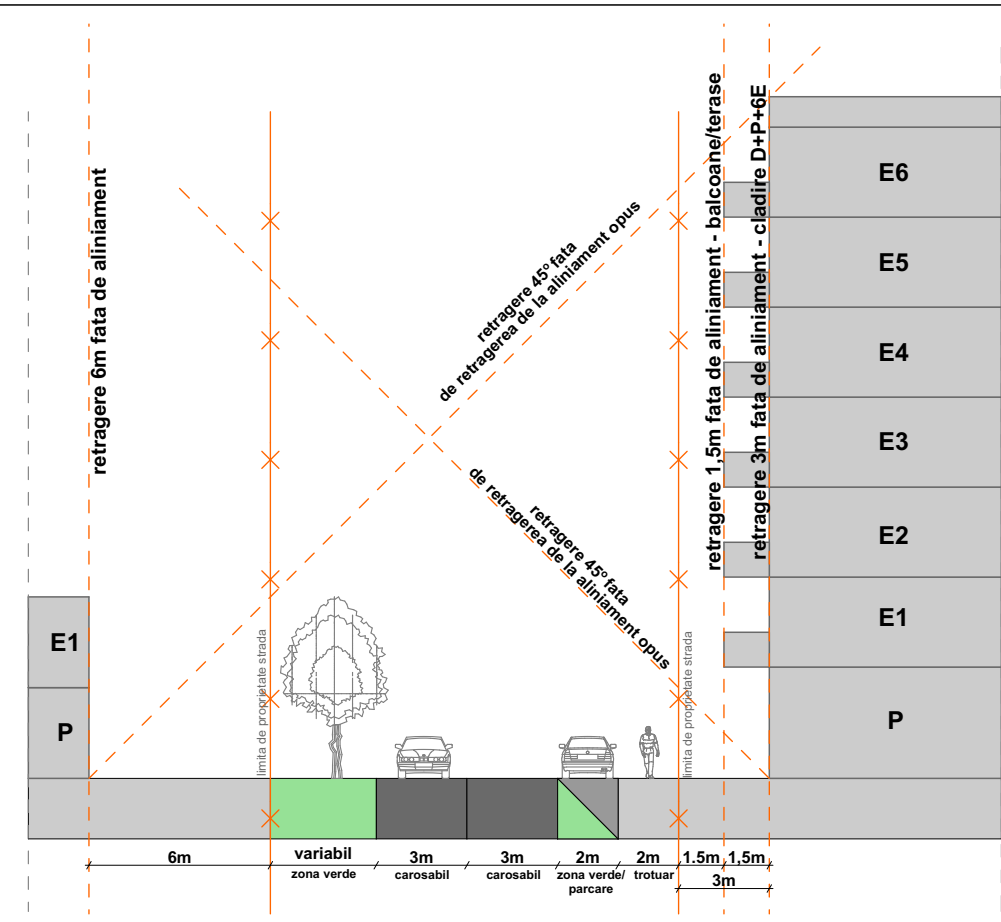
PROFIL STRALAL PROPUZ STR. LEGUMICULTURII SECTIUNEA 1-1
