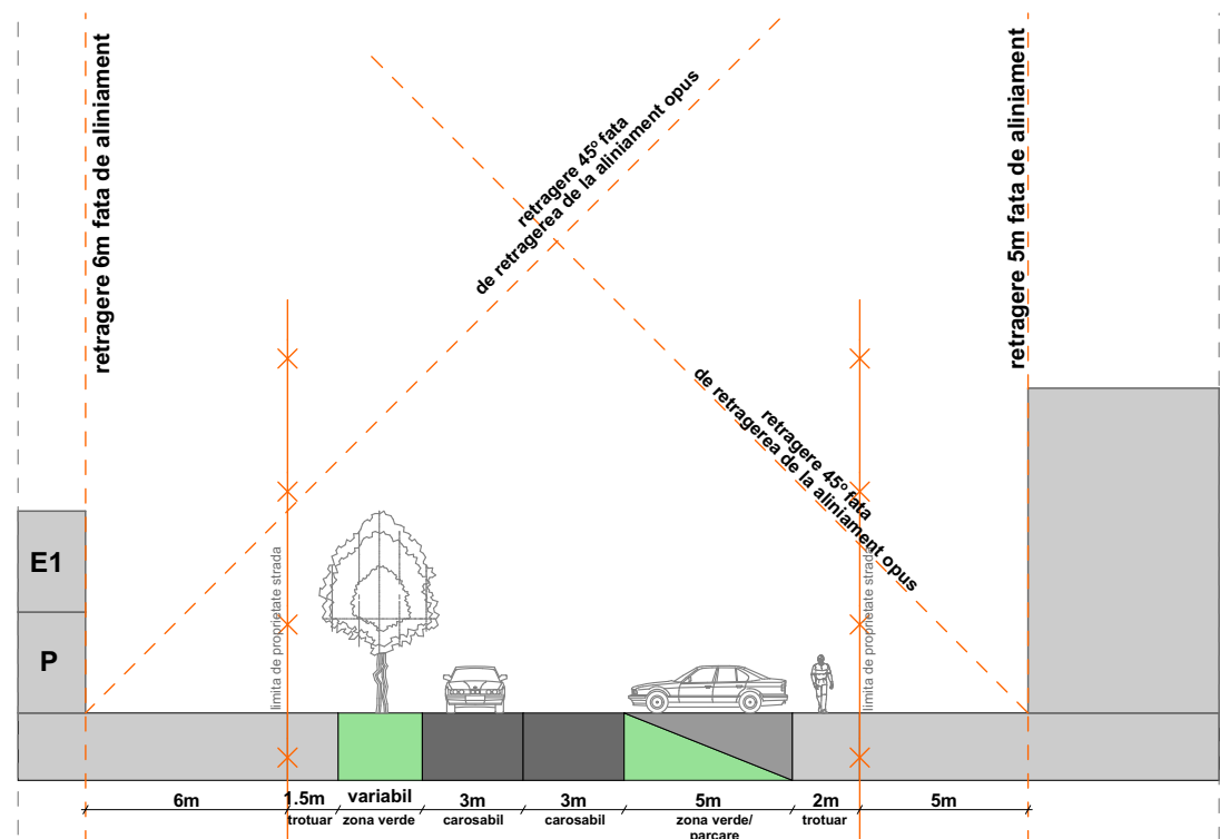
PROFIL STRALAL PROPUZ STR. LEGUMICULTURII SECTIUNEA 2-2
