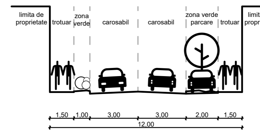
PT3 - Profil rezidențial - lățime 12 m
