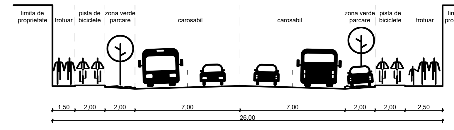
PT1 - Profil stradă colectoare cu infrastructură verde - lățime 26 m
