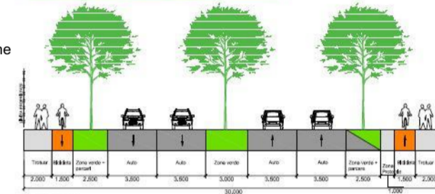
Profil transversal str. Constructorilor propus prin PUG aflat în curs de aprobare
